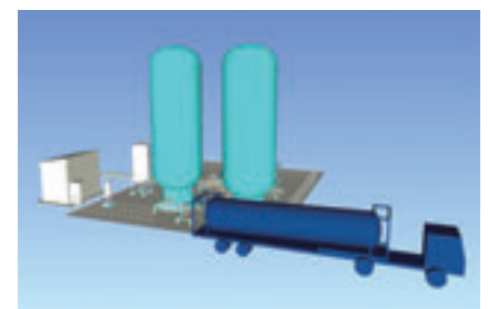
LNG 貯槽 × 2 基のレイアウト例
